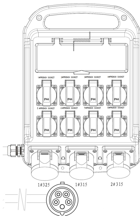
Obr. 1 Konstrukce rozvaděče
